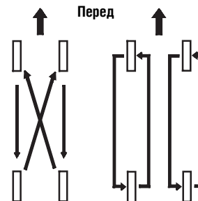
Шины с ненаправленным рисунком протектора
